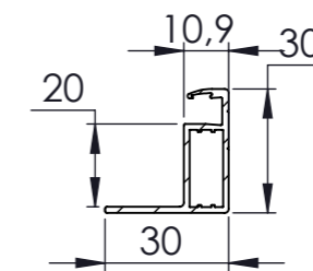
COUPE B-B ECHELLE 1 : 2
