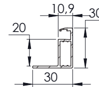
COUPE B-B ECHELLE 1 : 2
