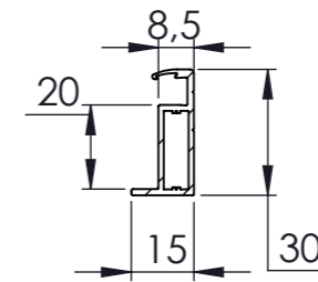
COUPE A-A ECHELLE 1 : 2
